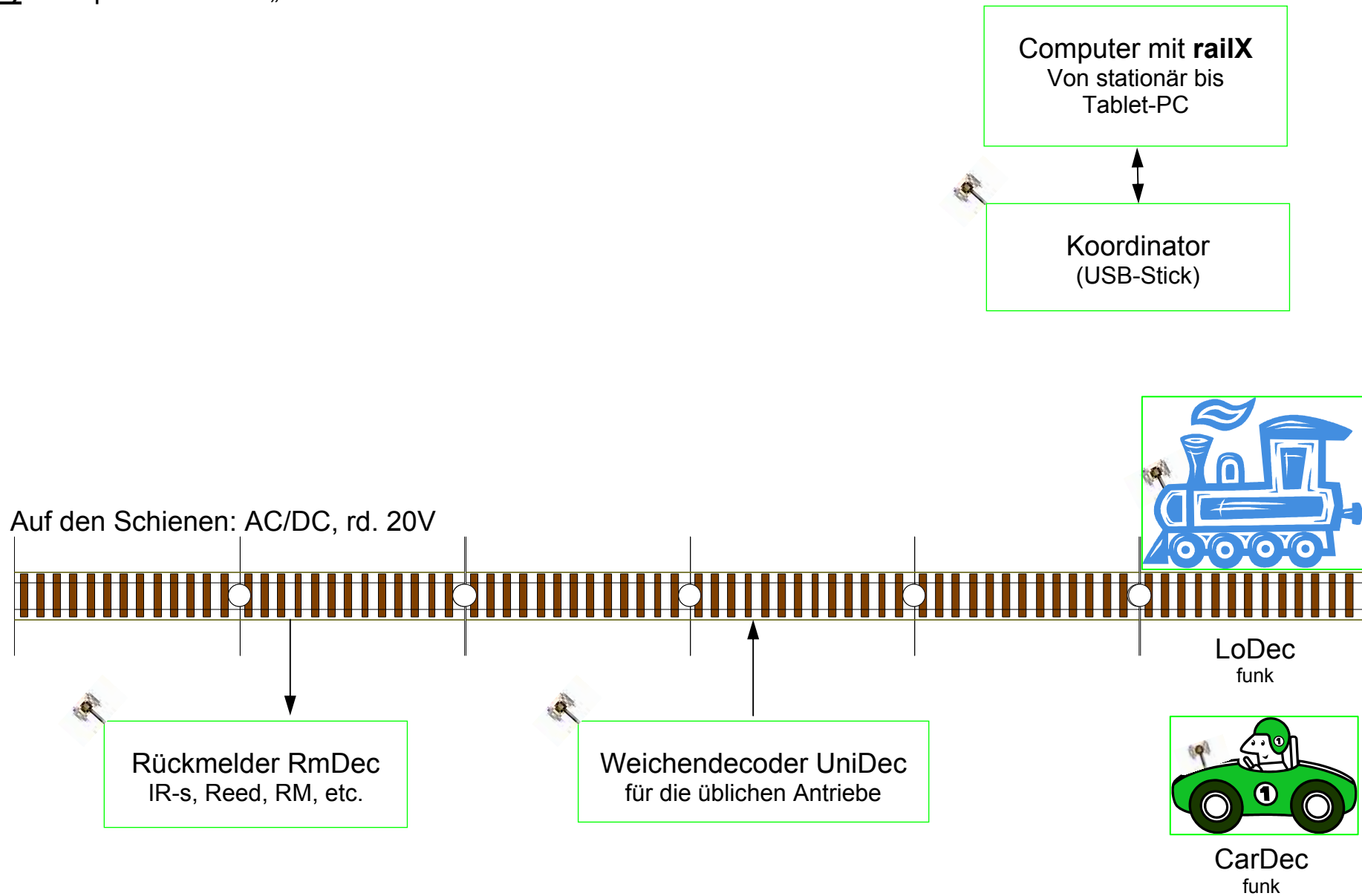
Fig. 2) Komponenten des „RailCommander“
