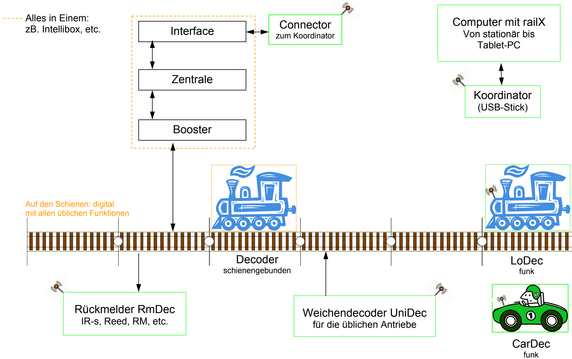
Fig. 4) Komponenten „RailCommander“ drahtlos inklusive Digitalsteuerung
